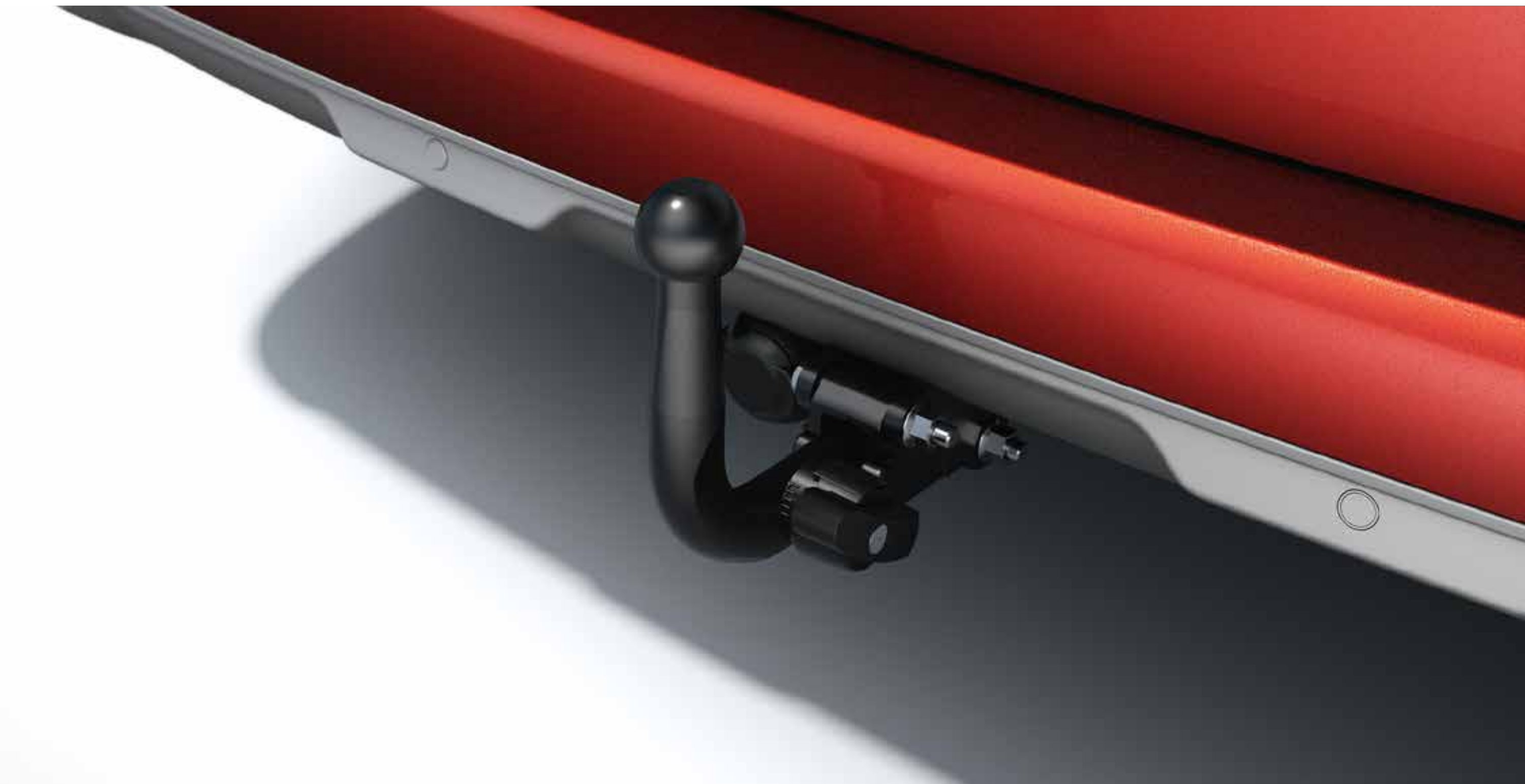
attelage RDSO Permet de tracter ou porter en toute sécurité remorque, bateau, caravane, matériel professionnel, porte-vélos... Démontable rapidement et sans outil, il devient invisible une fois la rotule enlevée.
